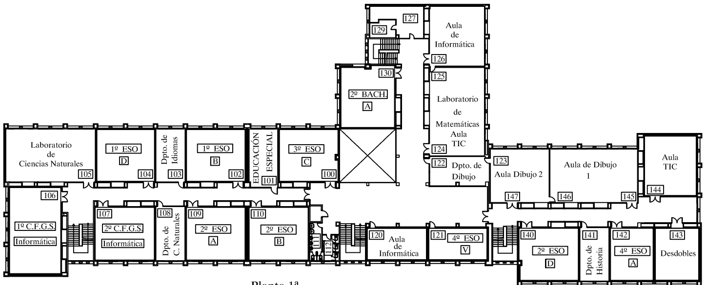
Planta 1ª
